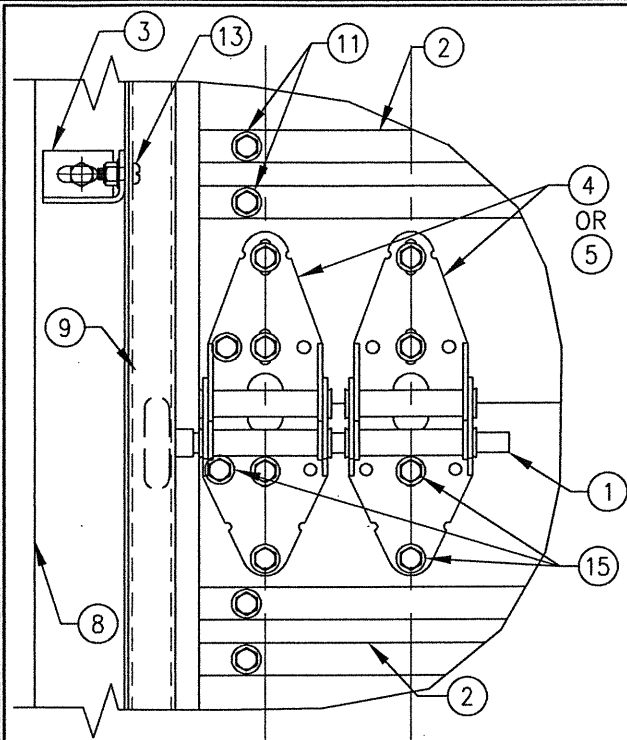
EDGE HINGE DETAIL
